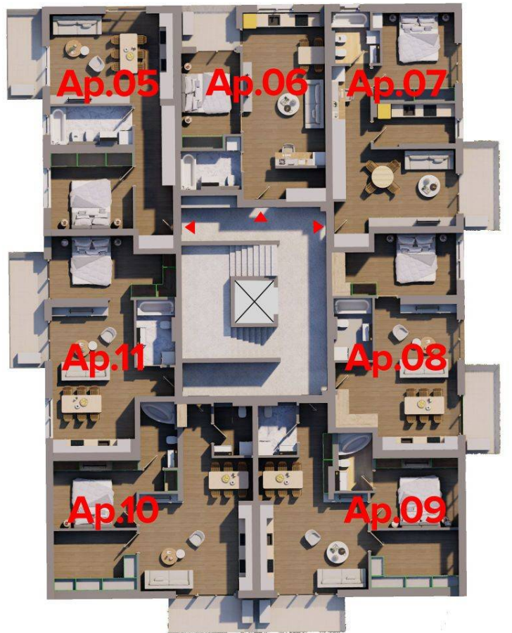
R37 PLAN ETAJ 1
